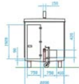
Heck offen
