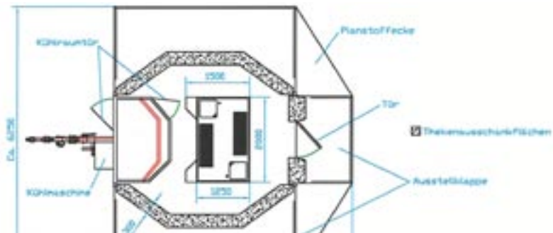
Draufsicht
