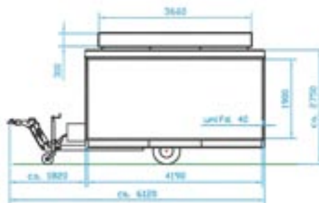
Seite geschlossen
